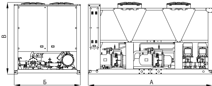
Габариты чиллеров LSA 250 - 1500
